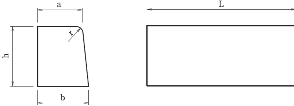
歩車道境界ブロック 片面
