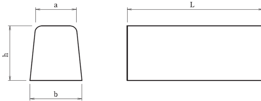
歩車道境界ブロック 両面
