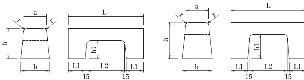
歩車道境界ブロック 両面 柵用
