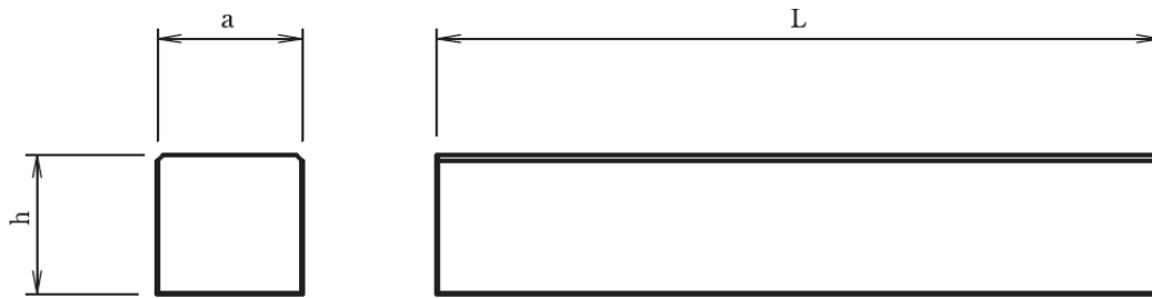
地先境界ブロック
