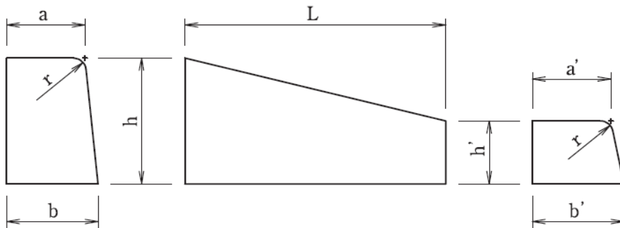
歩車道境界ブロック 乗入
