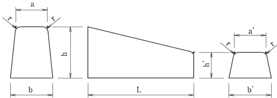
歩車道境界ブロック 両面 乗入
